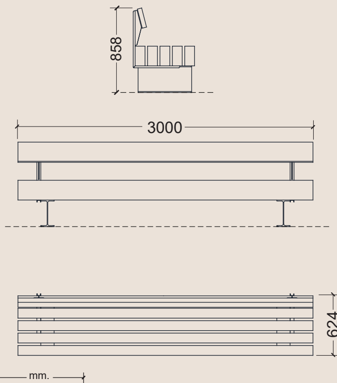
BANCO ZAIDIA (5 LAMAS) CON RESPALDO BENCH "ZAIDIA" (5 BEAMS WITH BACKREST) BANC "ZAIDIA" (5 BARRES) AVEC DOSSIER
