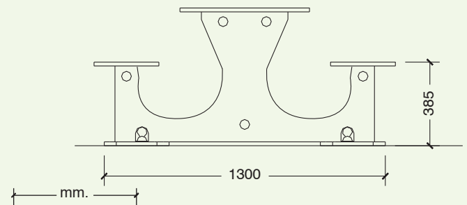
MESA INFANTIL 10 PLAZAS TABLE FOR KIDS (10 SEATS) TABLE POUR ENFANTS (10 PLACES)
