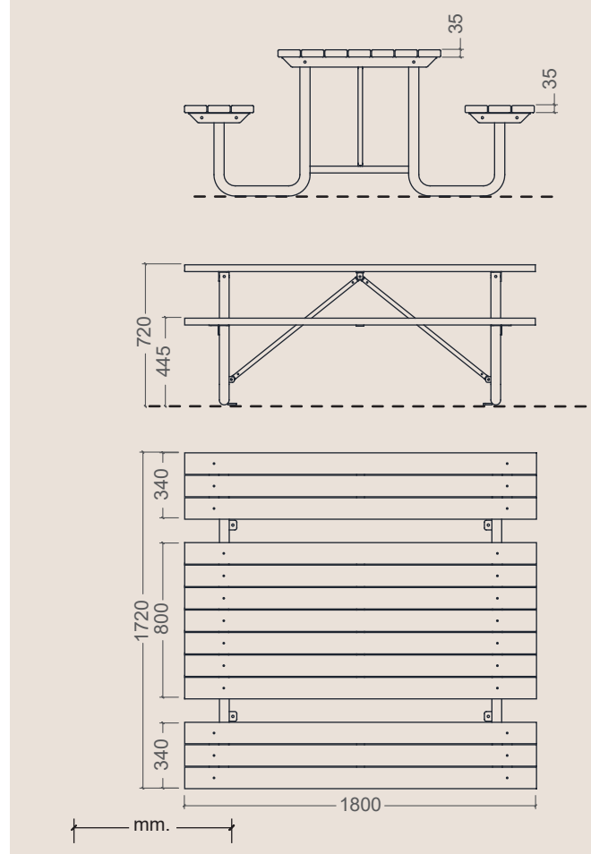
MESA CIUDAD (CON MADERA TÉCNICA) TABLE "CIUDAD" (WITH WPC) TABLE "CIUDAD" (AVEC BOIS COMPOSITE)
