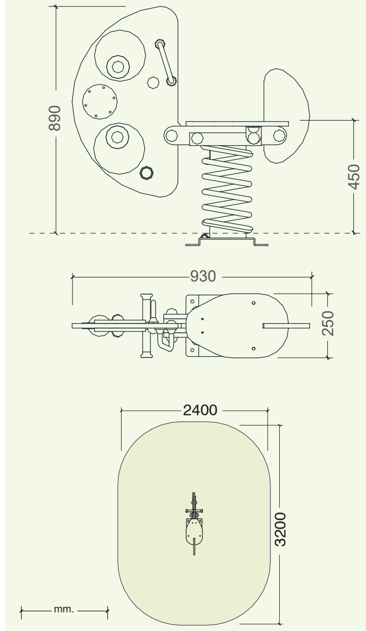
BALANCÍN DE MUELLES "MONSTER MONTY" SEESAW SPRINGER "MONSTER MONTY" JEU À RESSORT "MONSTER MONTY"
