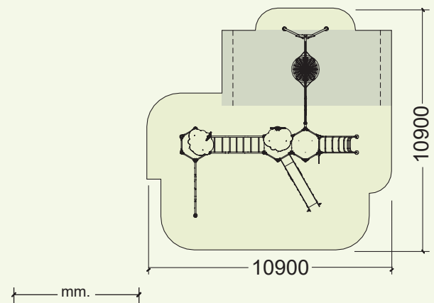
COMPLEJO "LA FRONDA" CON COLUMPIO CESTA COMBINATION "THE COPPICE" WITH NEST SWING COMBINAISON "LES BROUSSAILLES" AVEC BALANÇOIRE NID D'OISEAU
